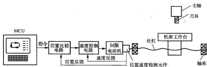
半闭环控制系统
