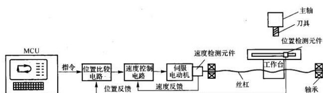
全闭环控制系统
